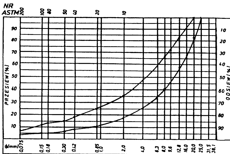
Rys. 1. Krzywe graniczne uziarnienia mieszanki mineralnej 0+25 mm do podbudowy z betonu asfaltowego dla KR 1-2
