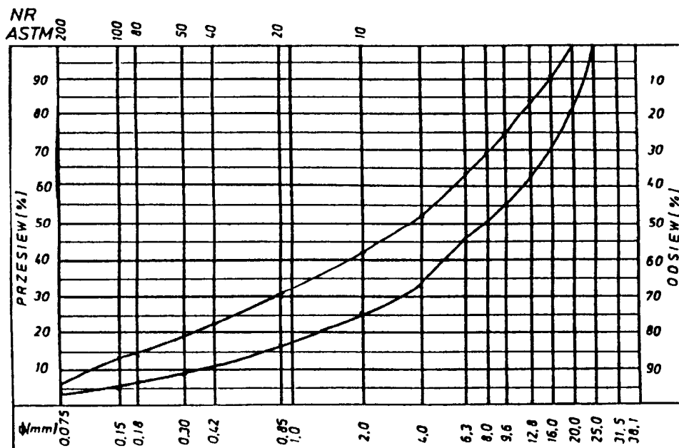
Rys. 11. Krzywe graniczne uziarnienia mieszanki mineralnej 0+25 mm do warstwy wiążącej, wyrównawczej i wzmacniającej z betonu asfaltowego dla KR 3-6(nie dotyczy)
