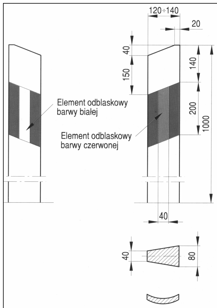
Wzór słupków prowadzących U-1a umieszczanych samodzielnie na poboczu
