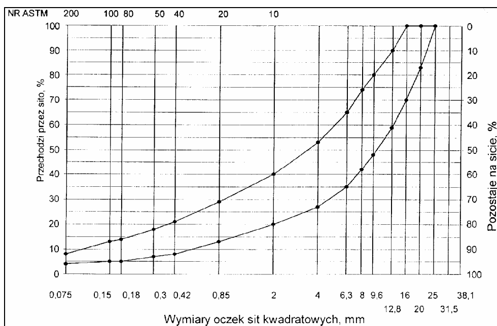
Rys. 1. Krzywe graniczne uziarnienia mieszanki mineralnej BA od 0 do 25mm do podbudowy nawierzchni drogi o obciążeniu ruchem KR 2
