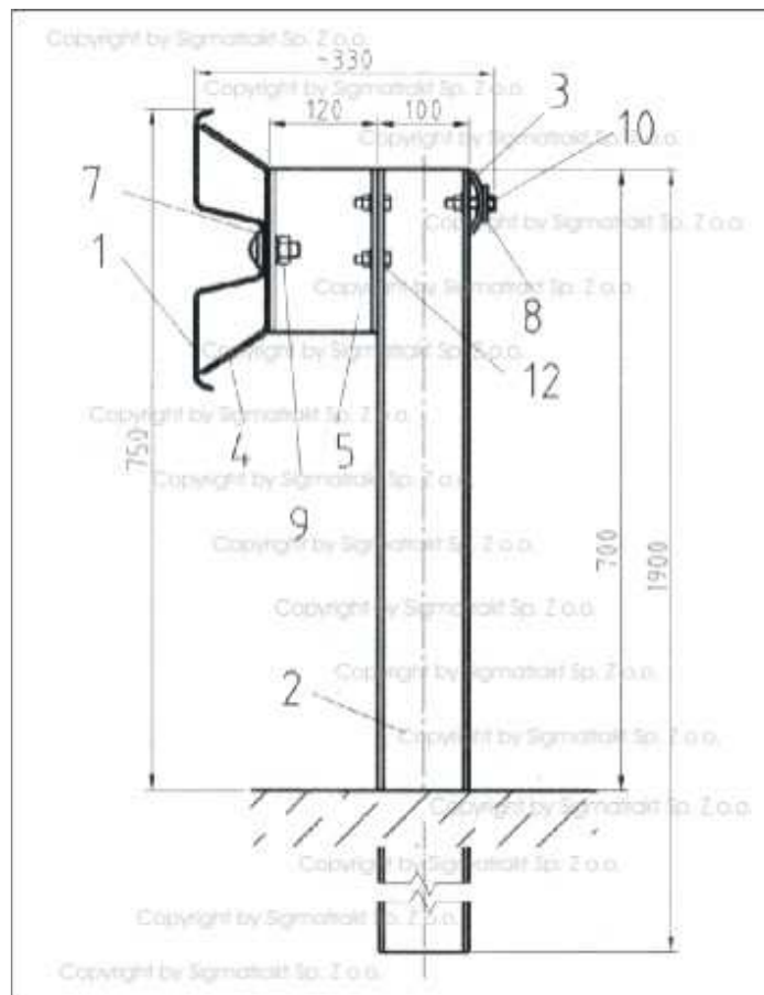
BARIERA SKRAJNA DROGOWA PRZEKŁADKOWA SP – 09/4 – ROZSTAW SŁUPKÓW CO 4m
